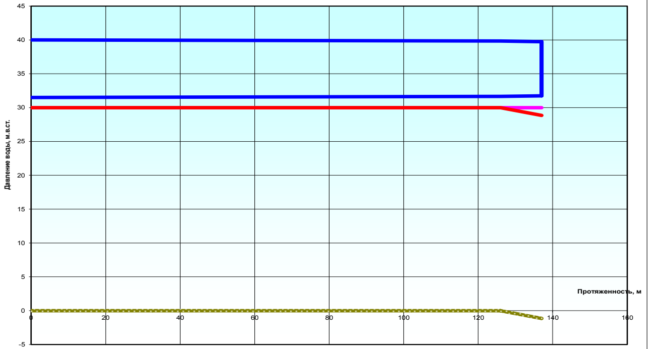
Пьезометрический график ( сетевая вода )
